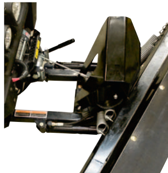
[ ELEKTRISCHE HYDRAULIKEINHEIT ]
